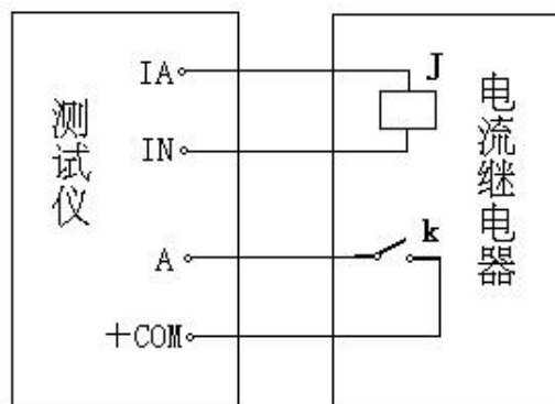
试验接线简图
