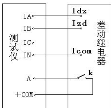
试验接线简图
